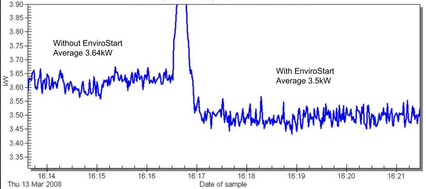
Denco, Hereford, UK 4kW Circ Fan
